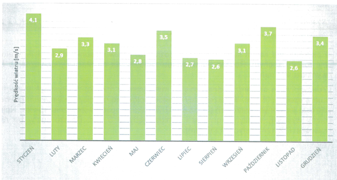
Rysunek 6 Przebieg średnich miesięcznych wartości prędkości wiatru w Płocku w 2025 r.
