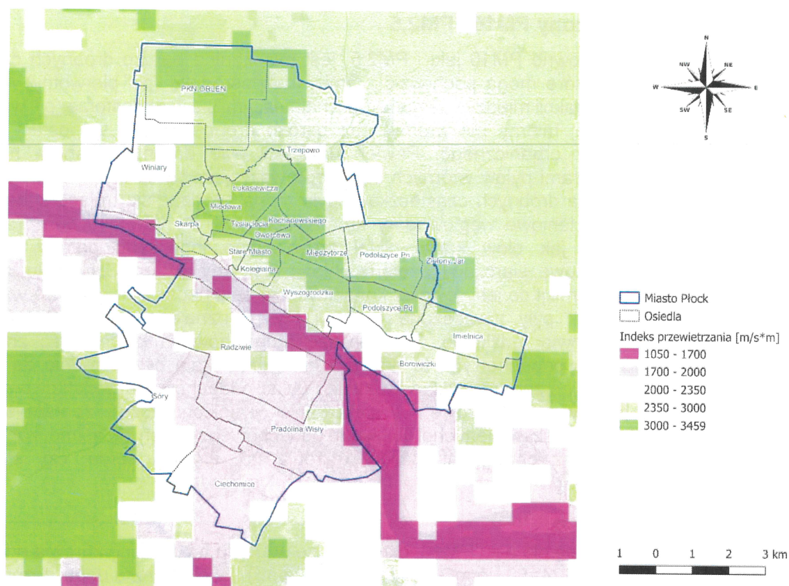
Rysunek 10 Indeks przewietrzania miasta Płocka w 2025 r.
