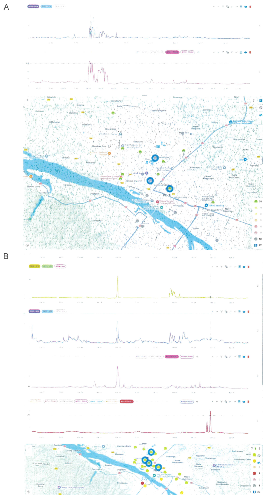
Rysunek 24 Wybrane epizody podwyższonych stężeń benzenu: A) na stacjach PMŚ w Płocku (GP52, GP53) w porównaniu do pomiarów wskaźnikowych stężeń odorowo-rafineryjnych na stanowisku WP21 (rondo Długa) oraz B) wyłącznie na dachu budynku Politechniki (WP25) z wizualizacją sytuacji wiatrowej
