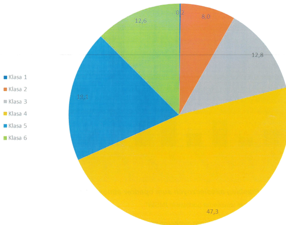
Rysunek 9 Udział klas równowagi atmosfery Pasquilla w Płocku w 2025 r.
